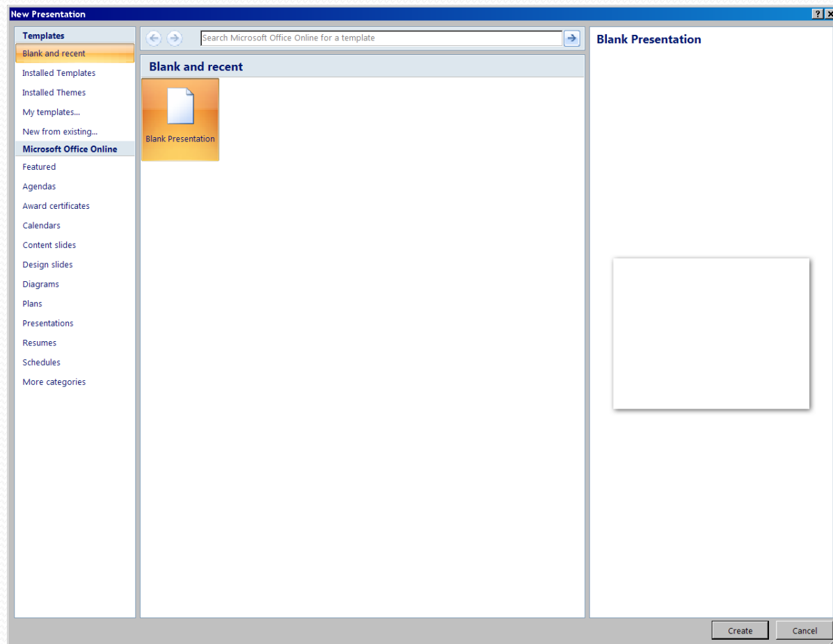
Slika 2. Kreiranje prezentacije
