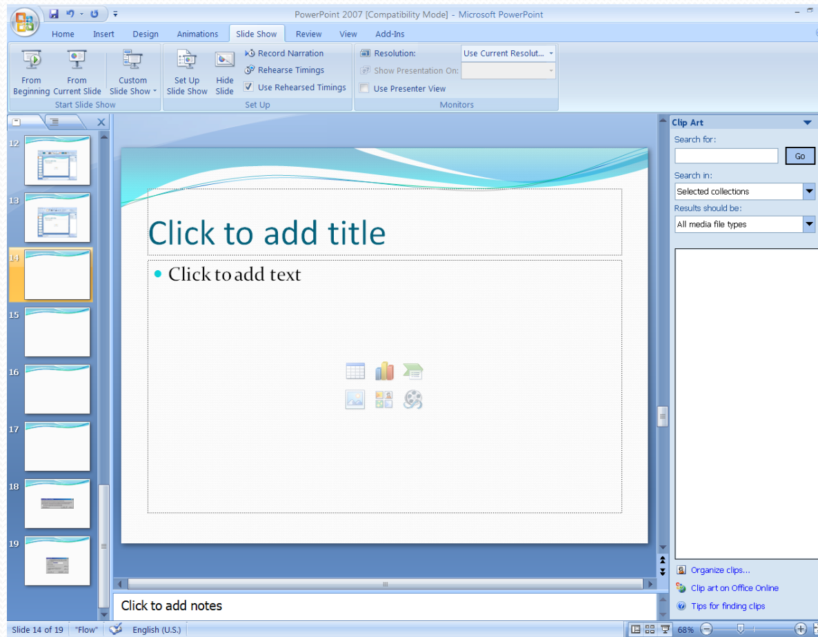
Slika 7. Slide Show
